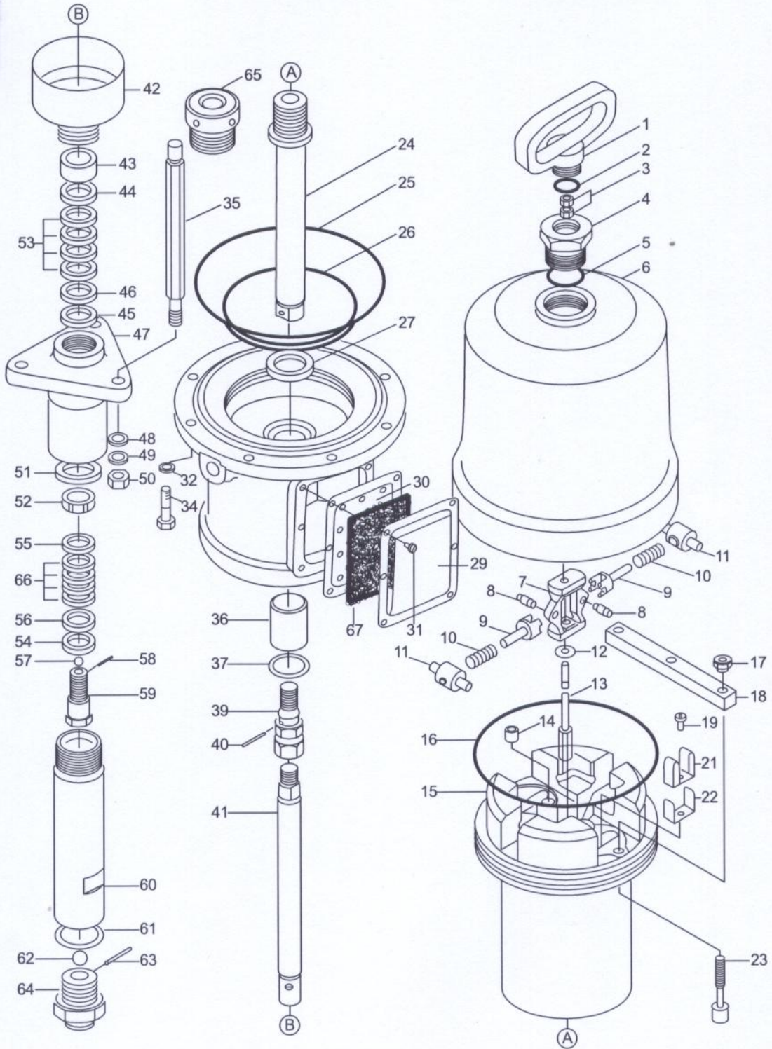
Pump Type PP 4301E
